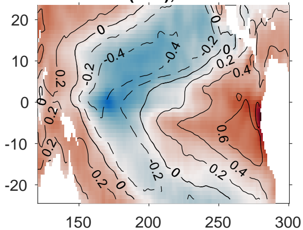
SVD2(SST); scf=0.06
