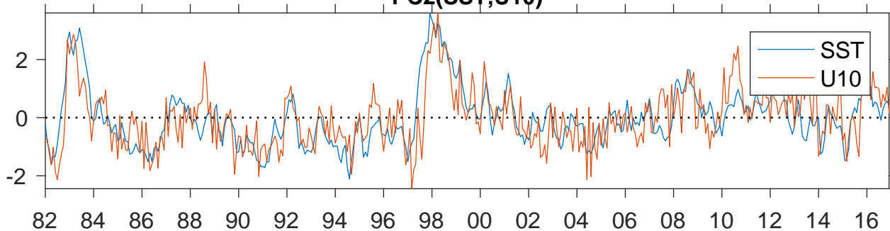
PC2(SST,U10)
