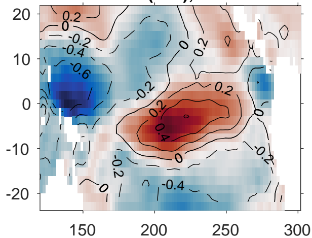
SVD2(U10); r=0.7
