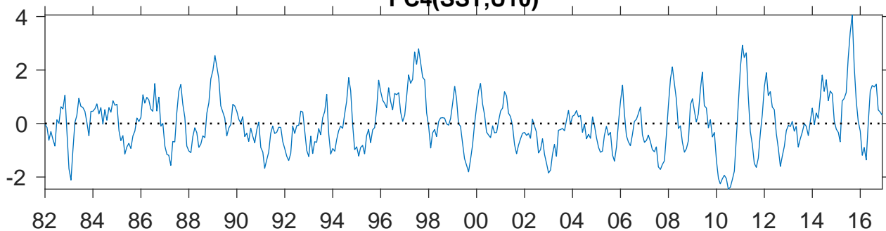
PC4(SST,U10)
