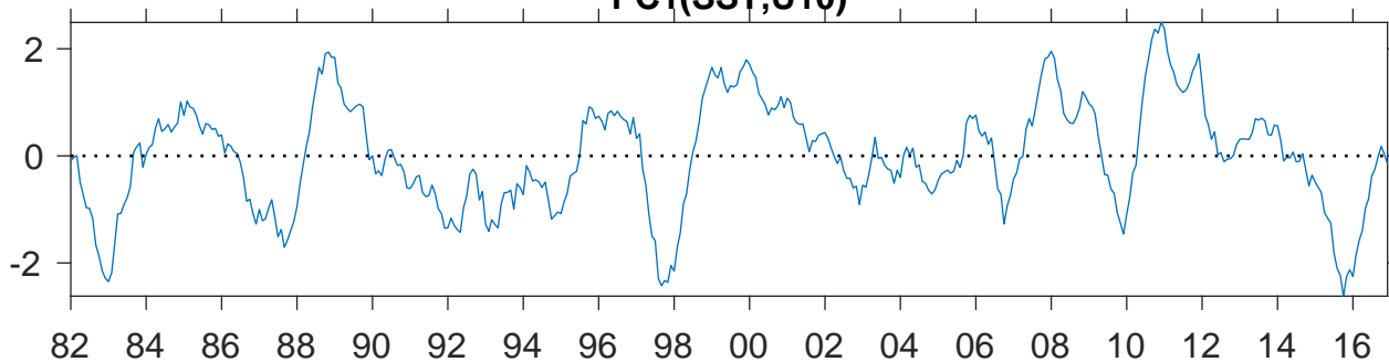
PC1(SST,U10)
