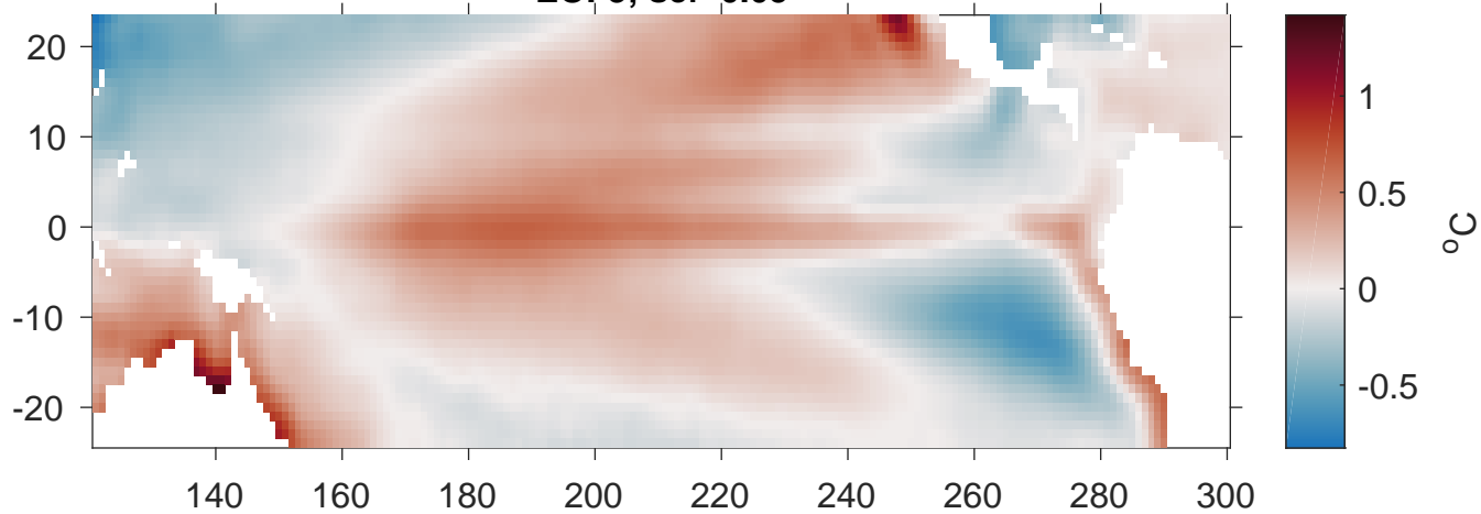
EOF3; scf=0.05
