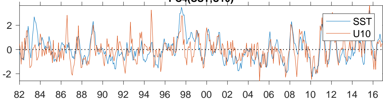
PC4(SST,U10)
