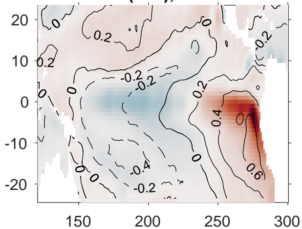
SVD4(SST); scf=0.03
