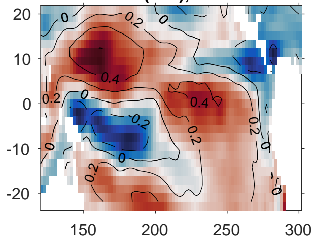
SVD4(U10); r=0.61
