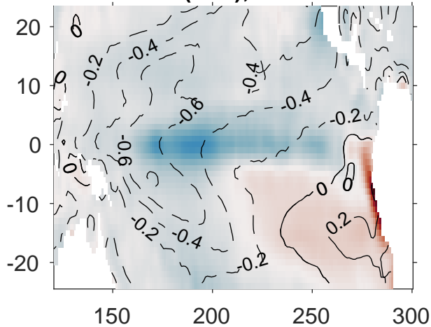
SVD3(SST); scf=0.08
