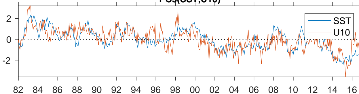
PC3(SST,U10)
