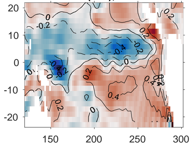
SVD3(U10); r=0.68
