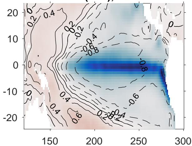
SVD1(SST); scf=0.7
