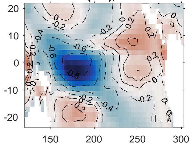
SVD1(U10); r=0.85
