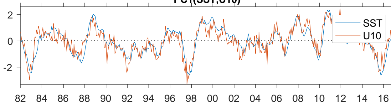
PC1(SST,U10)
